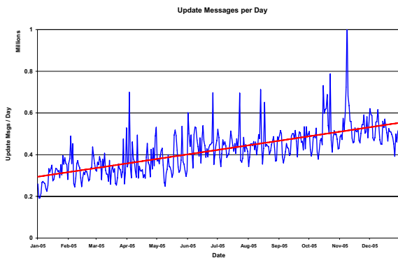
Figure 1. BGP Update messages per Day
